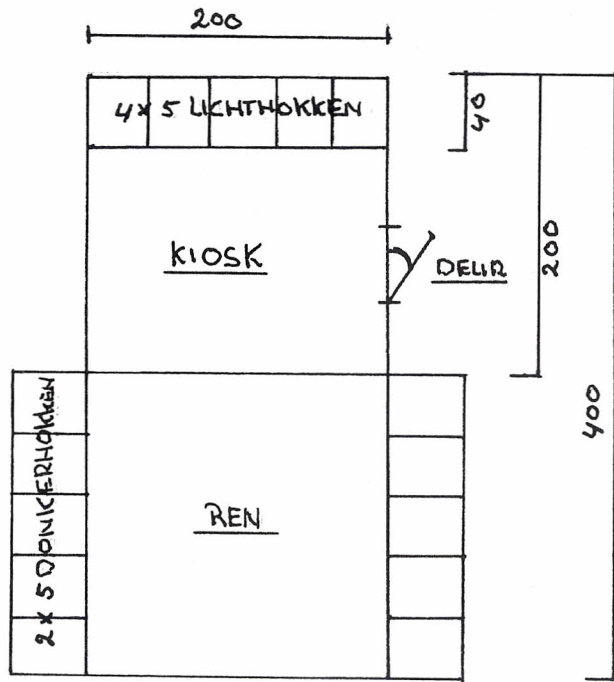
BOVEN - AANZICHT
