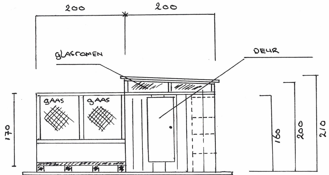
ZIJ - AANZICHT
