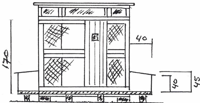
VOOR - AANZICHT
